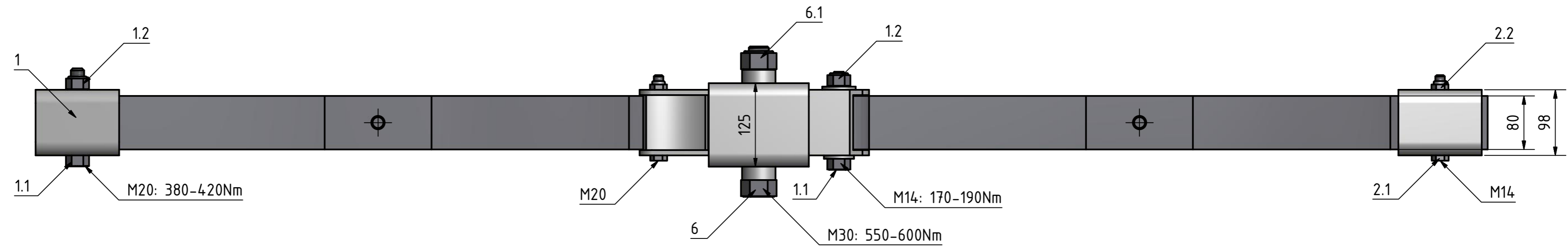
Übersicht Parabelfederaggregate
